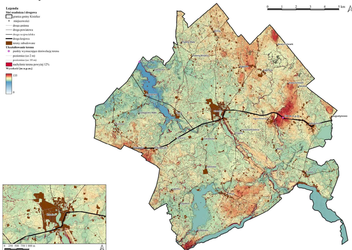
Rysunek 16. Ukształtowanie terenu na obszarze gminy Kisielice.
