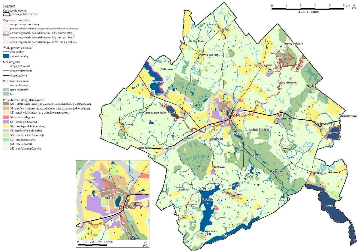
Rysunek 26. Zagrożenie powodzią na terenie gminy Kisielice na tle projektowanych stref planistycznych. Źródło: Opracowanie własne.
