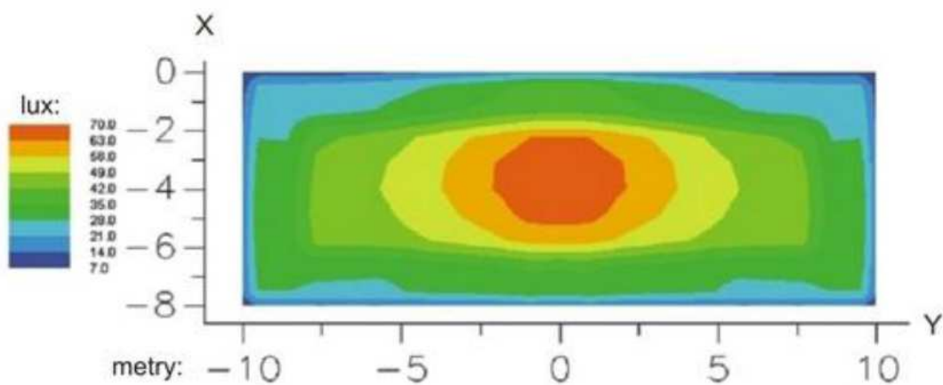
Rys. 6. Rozkład oświetlenia dla drogowej lampy sodowej (250W)
