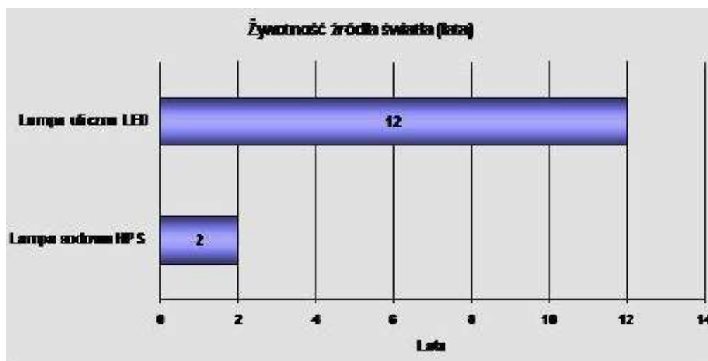
Rys. 4. Żywotności lamp sodowych (HPS) i lamp Power LED
