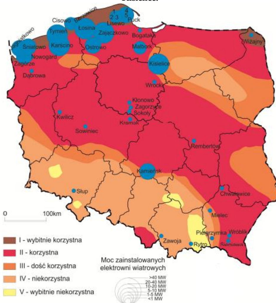
Rysunek 8. Strefy energetyczne wiatru wg H. Lorenc z uwzględnieniem położenia gminy Kiszelice.
